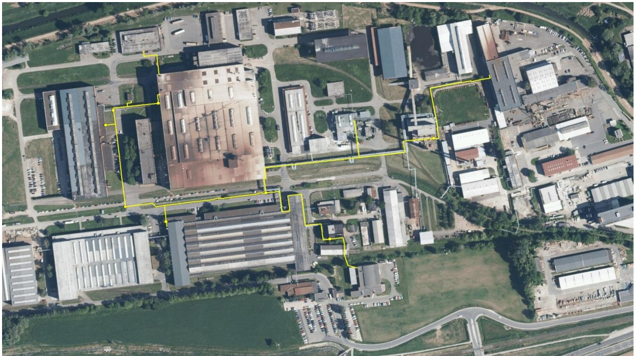
Schéma rozvodů zemního plynu LDS Local Energies, a.s.
